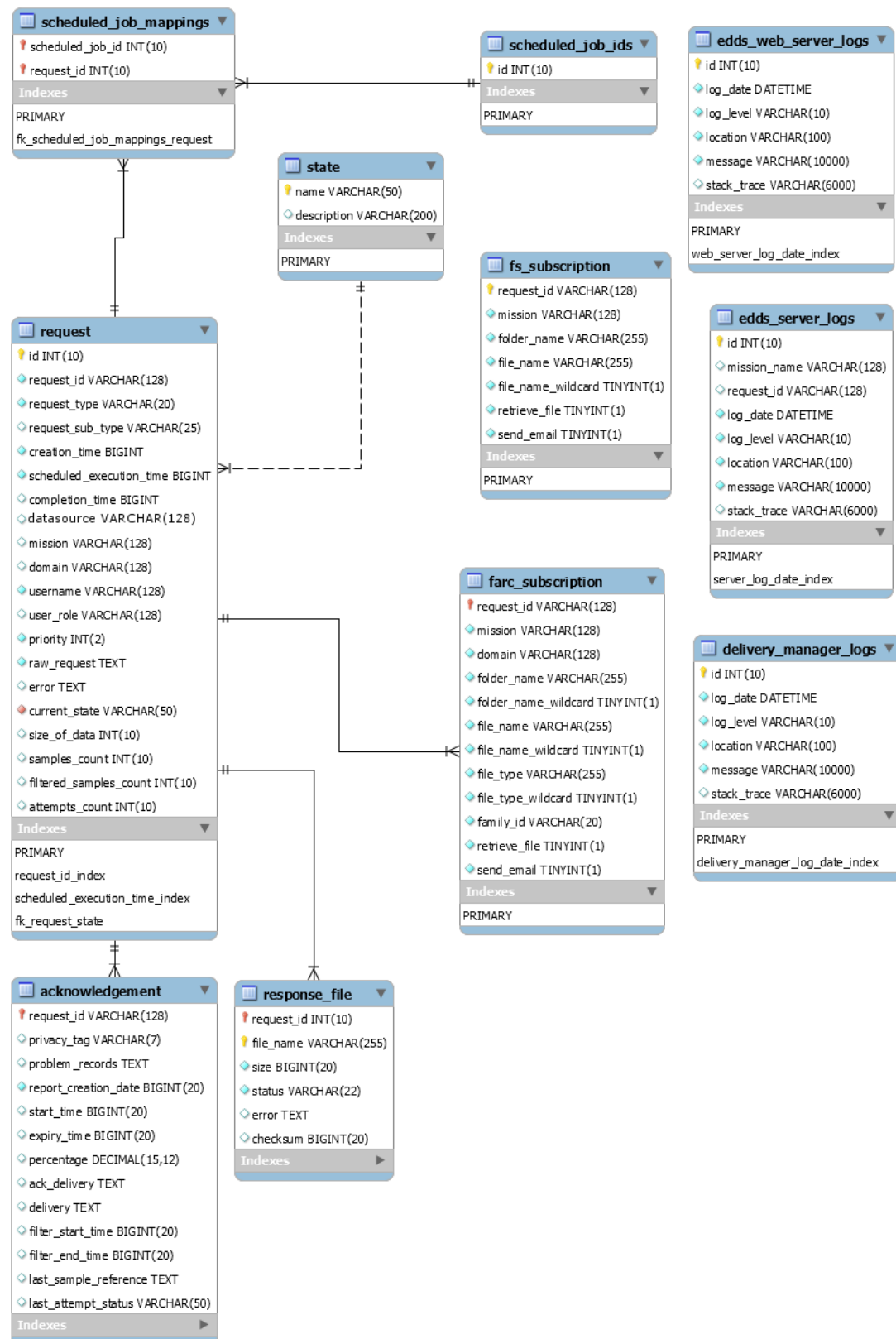
Figure 39 - database ER diagram
